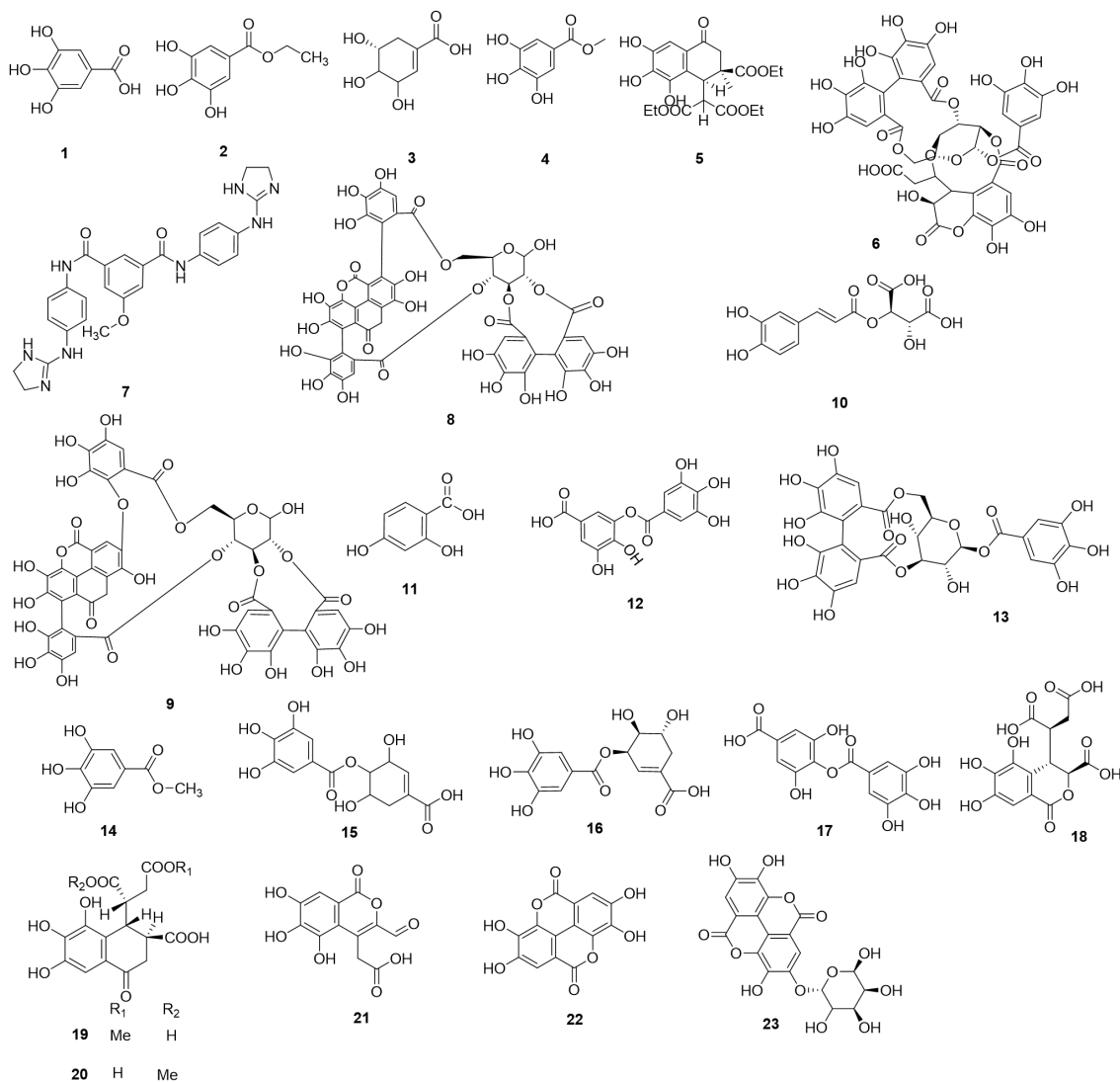
图 1 化合物 1~23 的化学结构
