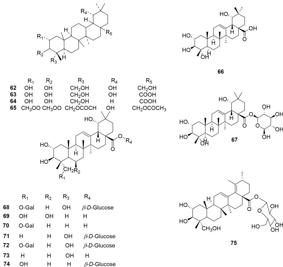
图2 化合物 62~74 的化学结构
