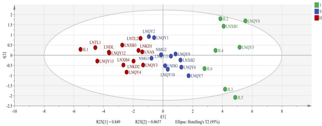
图 4 OPLS-DA 得分图
