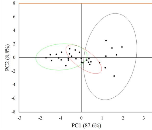
图 3 PCA 得分图
