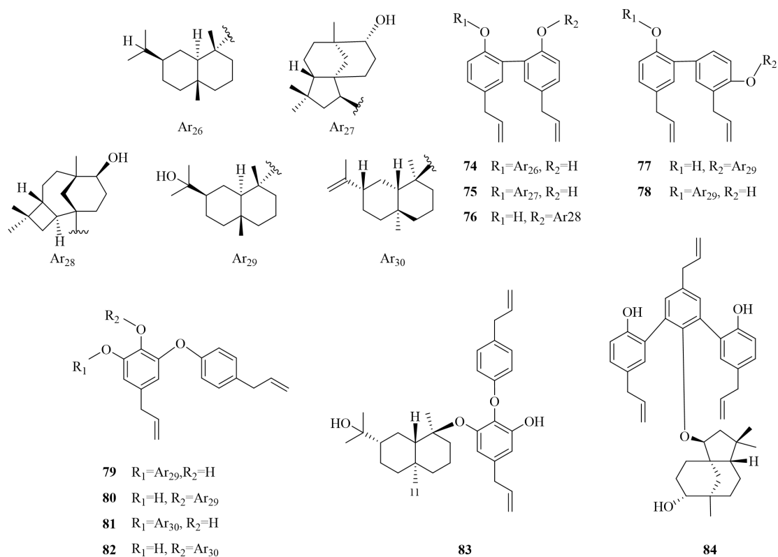
图 3 天然倍半萜木脂素的化学结构
