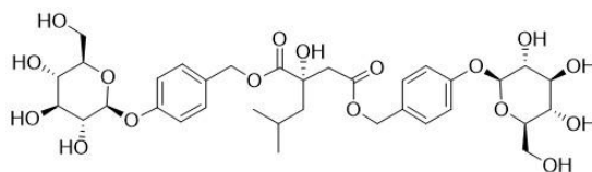
图 1 Militarine 的化学结构
